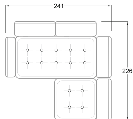
Kleine Ecke mit 1 Arm- und 4 Rückenlehne 1xFS-1xES-4xLR-1xLN
